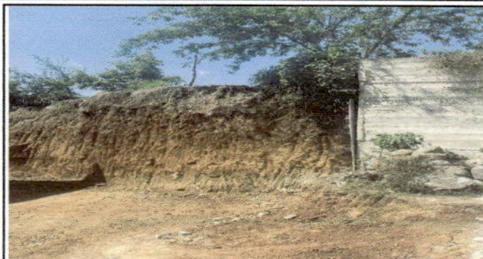
Foto 2: Reparación de muro de contención EORM del Paraje El Pito, Aldea Subchal.
