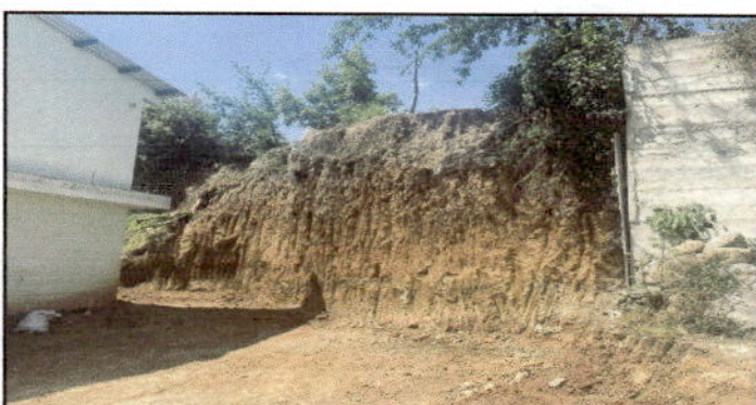
Foto 6: Reparación de muro de contención EORM del Paraje El Pito, Aldea Subchal.
